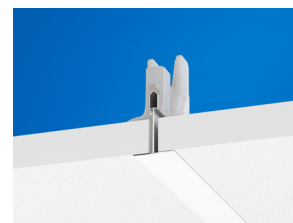
Connect T24 Hovedprofil C4 med Connect Hygiene Clip
