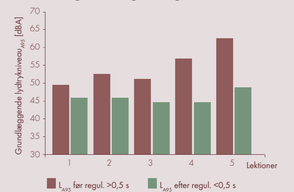
Aktivitetslydniveauer ( L_{A95} ) før og efter regulering 3
